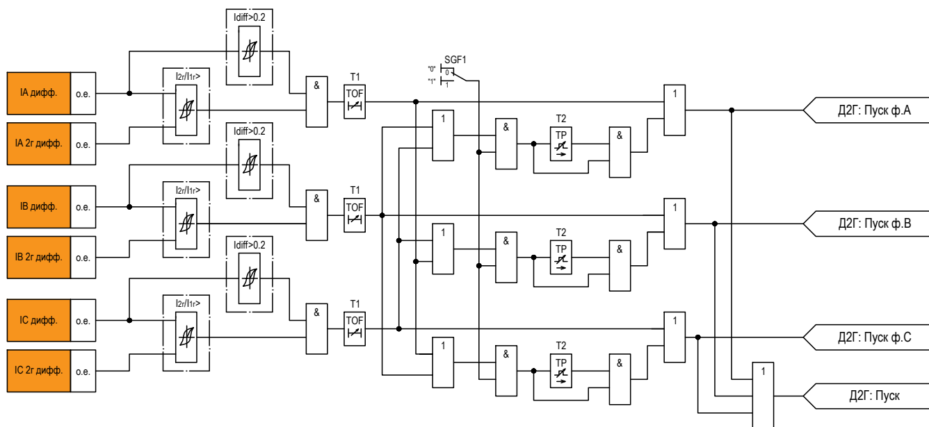
Рисунок 2.5 – Функциональная схема логики Д2Г
