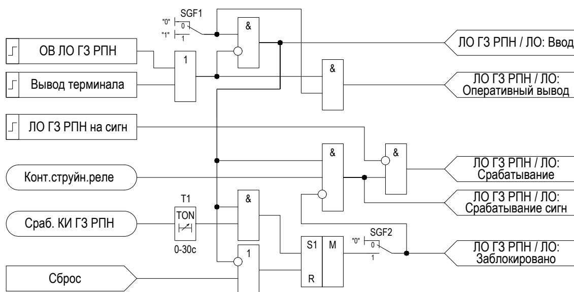
Рисунок 2.20 – Функциональная схема логики отключения при срабатывании струйного реле РПН трансформатора
