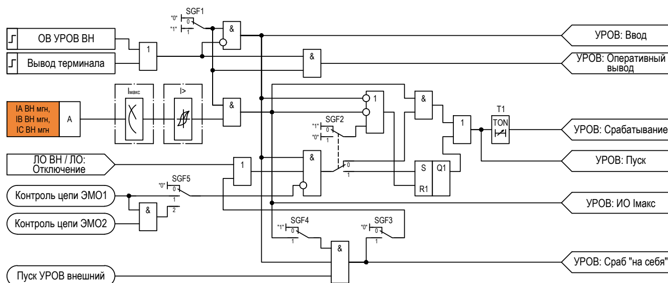
Рисунок 2.31 – Функциональная схема логики УРОВ
