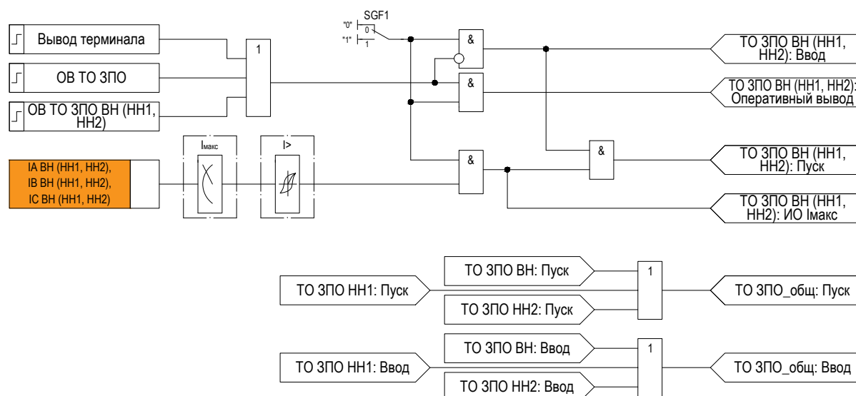
Рисунок 2.13 – Функциональная схема логики ТО ЗПО
