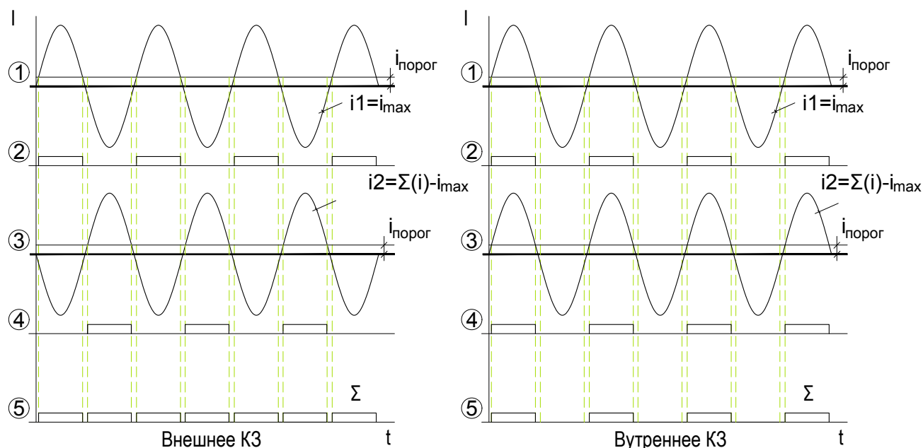
Рисунок 2.7 – Временные диаграммы работы БВКЗ
