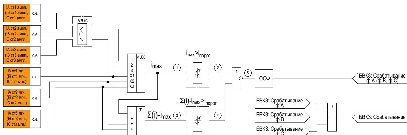
Рисунок 2.8 – Функциональная схема логики БВКЗ
