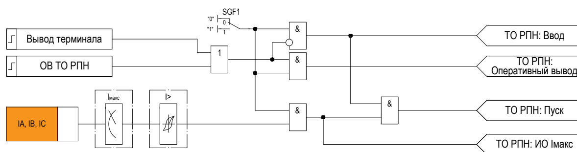
Рисунок 2.17 – Функциональная схема логики ТО РПН
