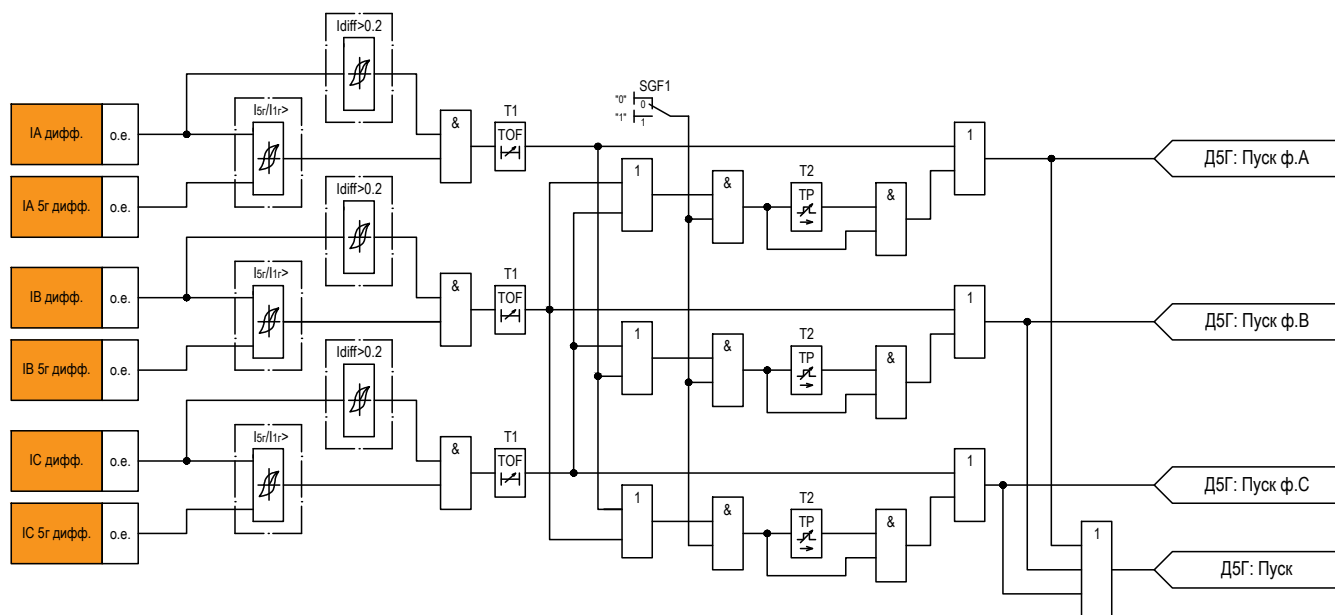
Рисунок 2.6 – Функциональная схема логики Д5Г
